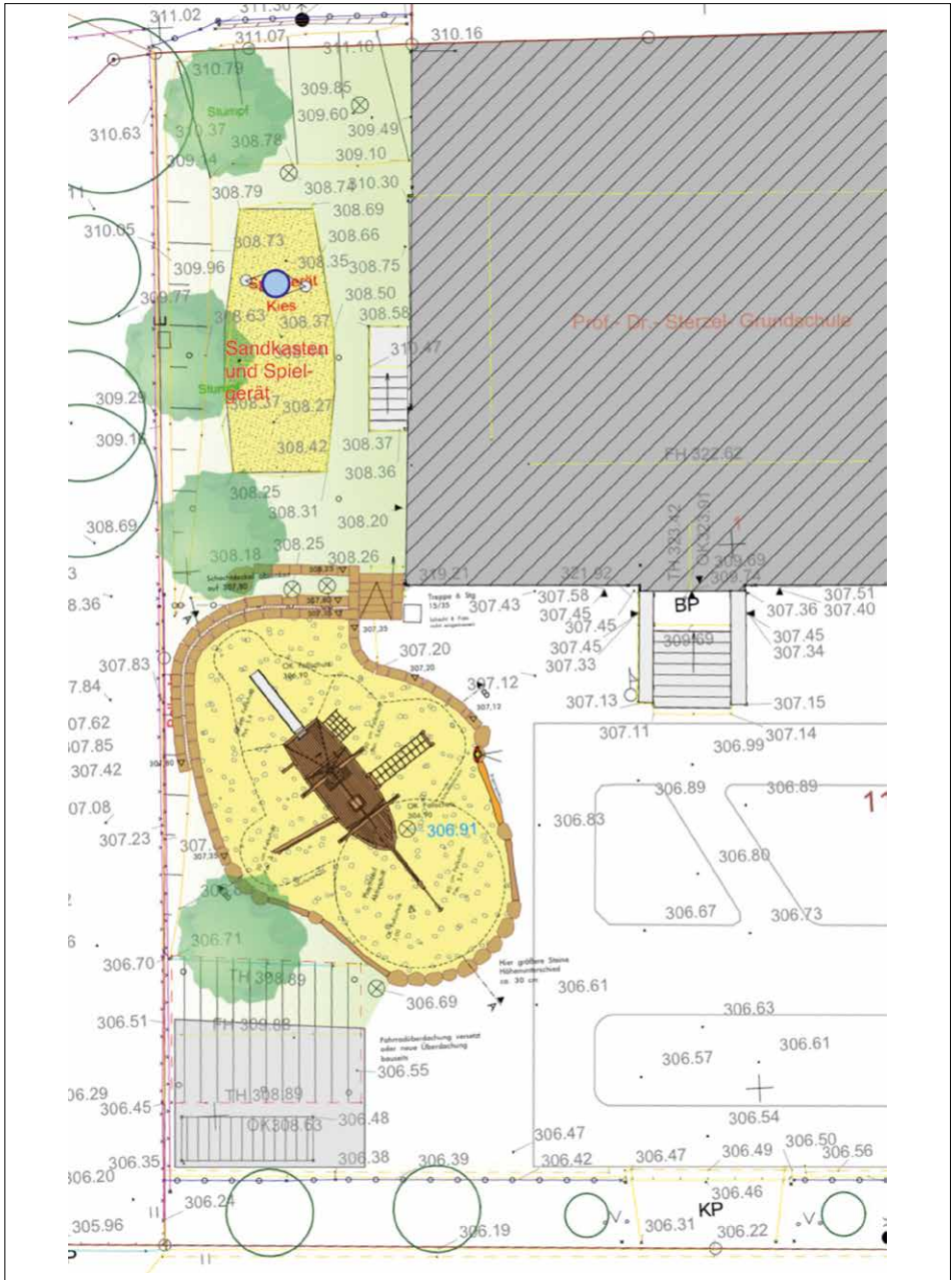
Planungsentwurf Schulhof
